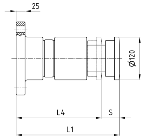
Ausführung FF
