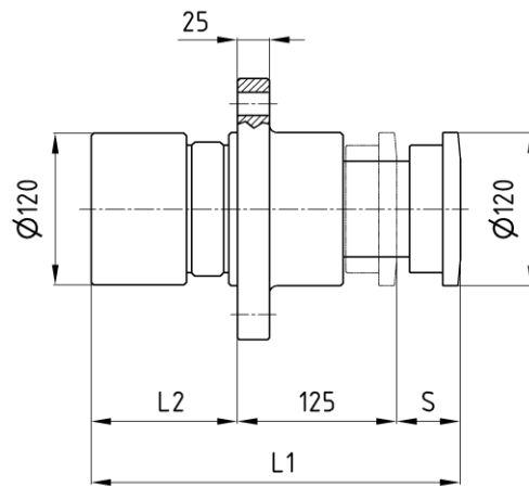
Ausführung EF
